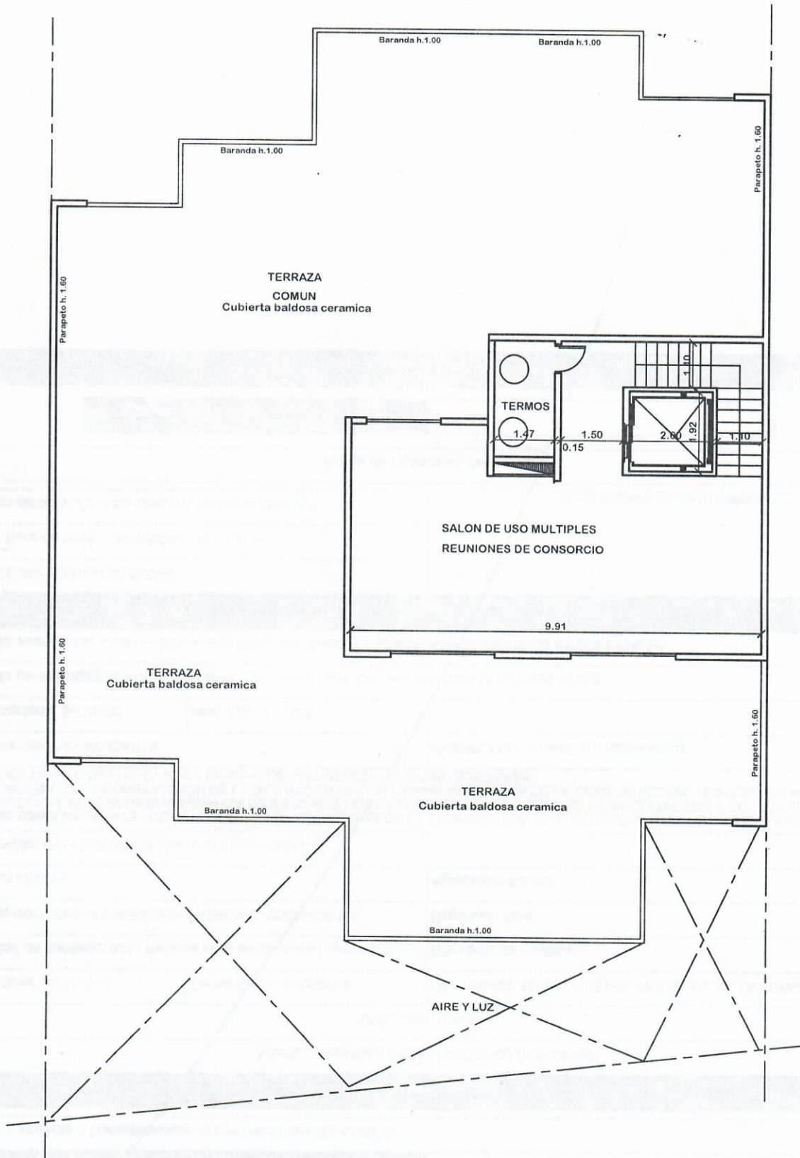
PLANTA AZOTEA
